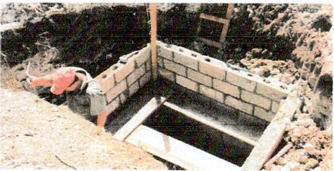
Foto 3: Mejoramiento de sanitarios y migitorio con pared de block
